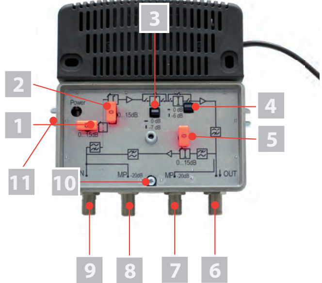
Bild 2: Verstärker HV 432, Innenansicht (HV 433, HV 431 und HV 331 ähnlich)
